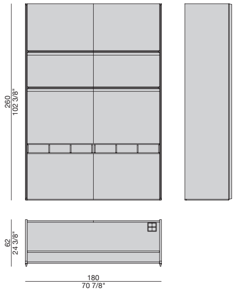
Modulo scrittoio 180 Writing desk module 180
