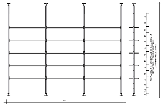
COMP. U46
