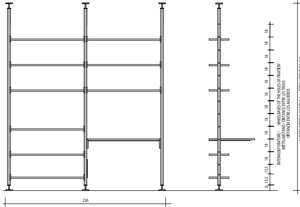
COMP. U33
