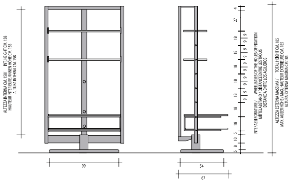
COMP. U27
