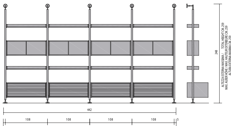
COMP. U51
